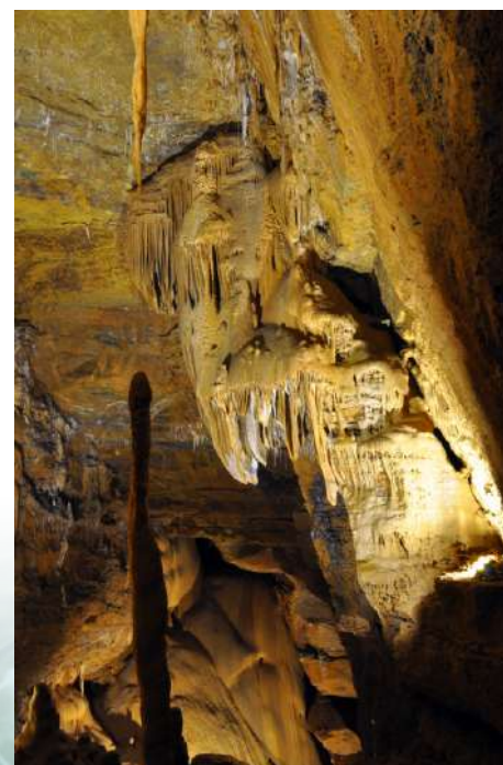
Stalactite - Stalagmite
